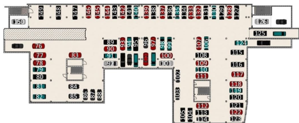
Схема расстановки автомобилей на подземном этаже №2 (отм. - 8.15) автопарковки по ул. Краснодарская, 8 Г, пом. 1
